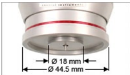
Durômetro Shore HPSD
