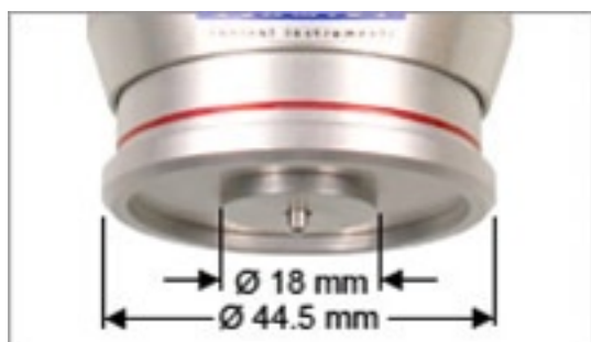
Durômetro Shore HPSDO
