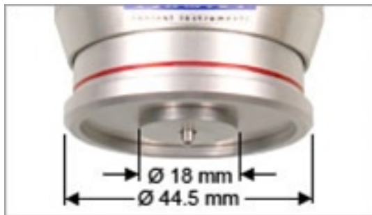
Durômetro Shore HPSO
